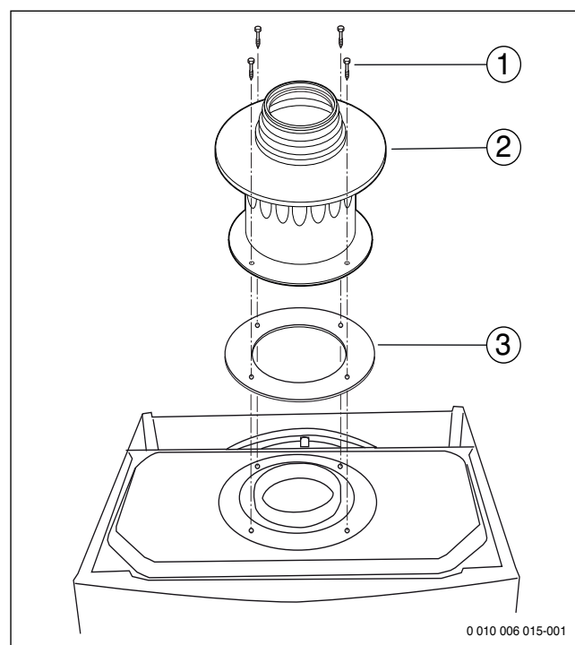
Рис. 18 При вертикальном отводе дымовых газов B_{22} и мощности котла = 35 кВт: установите переходник и дроссельную диафрагму
