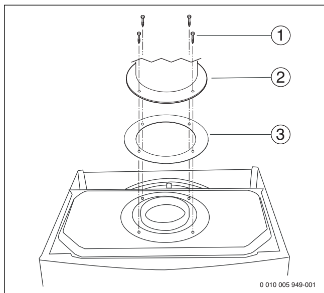
Рис. 16 Крепление переходника
